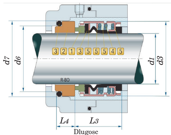
Pojedyncze uszczelnienie mechaniczne R-502
