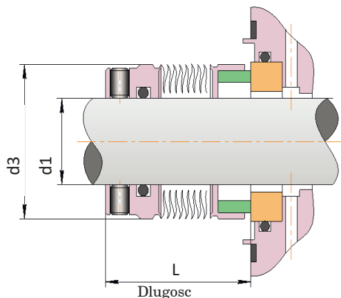
Uszczelnienie mechaniczne R-680 (676 / 670 / 680)
