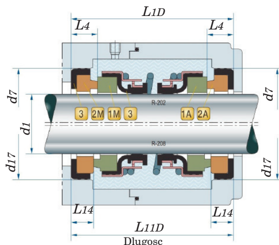
Dwustronna uszczelka mechaniczna R-202/R-208
